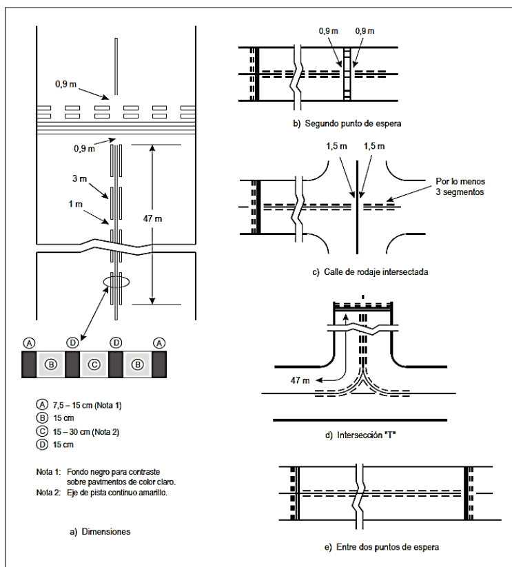
Figura 5-7. Señal mejorada de eje de calle de rodaje
