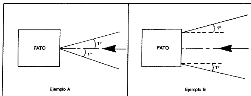
Figura 5-11H. Divergencia del sector “derrota correcta”
