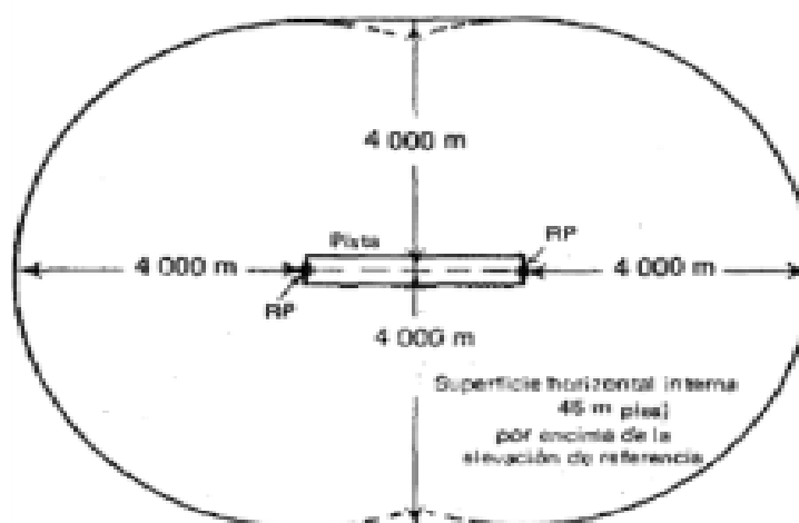
Figura 1. Superficie horizontal interna
