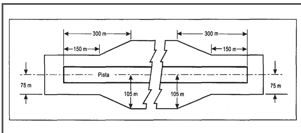
Figura A – 3. Parte nivelada de la franja de una pista para aproximaciones de precisión cuyo número de clave sea 3 ó 4.
