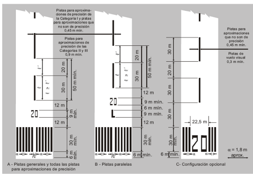
Figura 5-2. Señales de designación de pista, de eje y umbral
