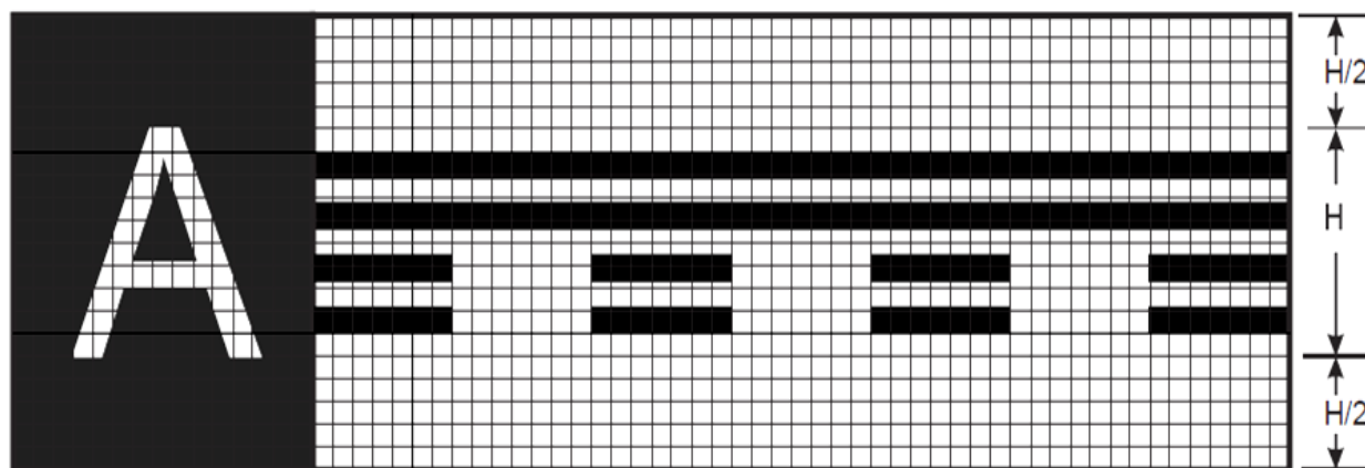
Letrero de pista libre (con el letrero típico de emplazamiento)
