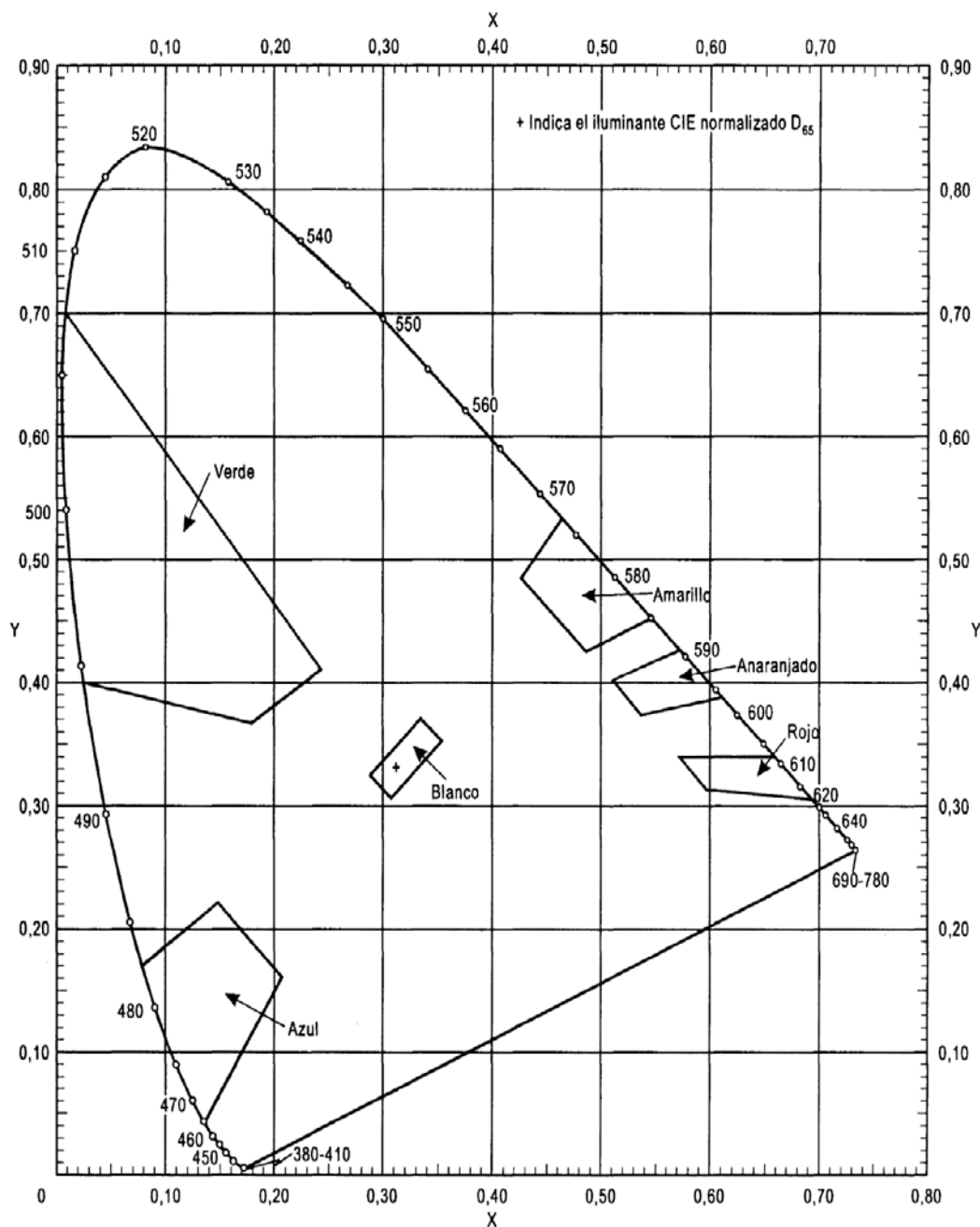
Figura A1 - 3. Colores de los materiales retrorrefletantes para las señales, letreros y tableros
