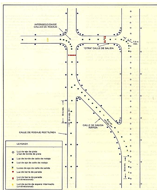
Figura 5-24. Luces indicadoras de calle de salida rápida
