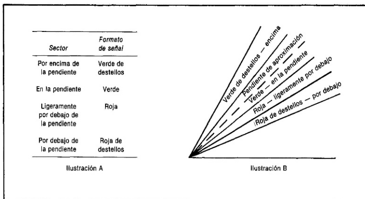
Figura 5-12H. Formato de la señal HAPI
