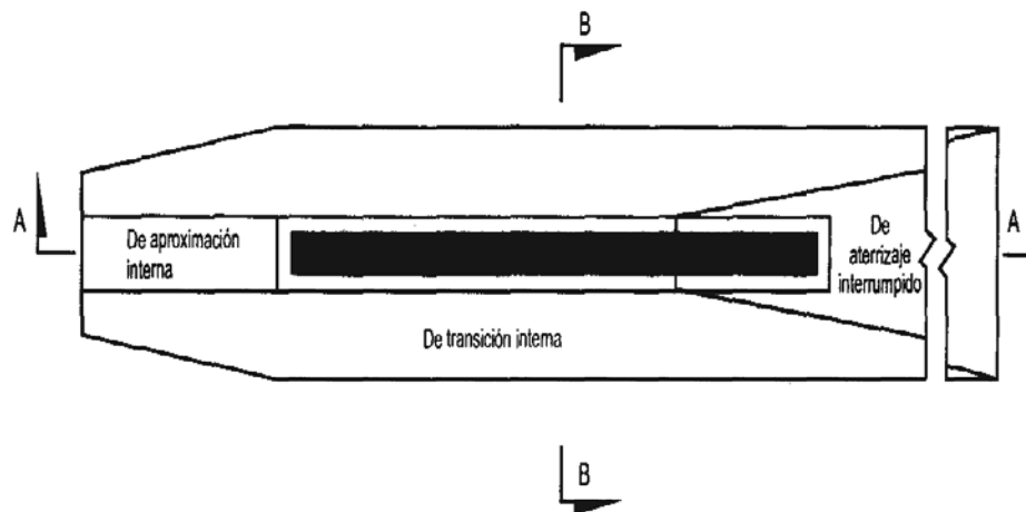
Figura 4.2. Superficies limitadoras de obstáculos de aproximación interna, de transición interna y de aterrizaje ininterrumpido
