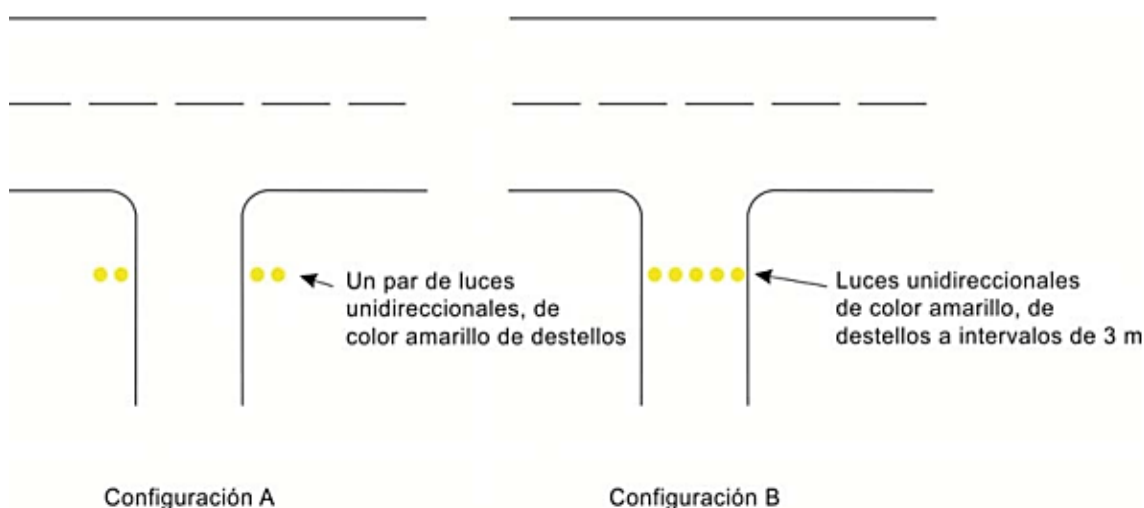
Figura 5-27. Luces de protección de pista
