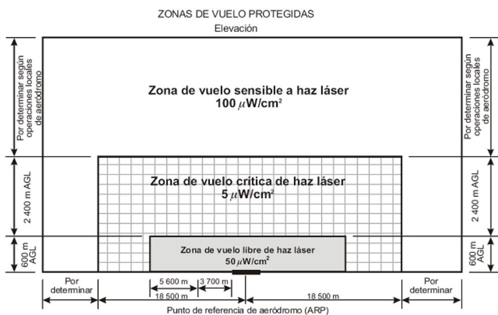
Figura 5-12. Zonas de vuelo protegidas indicando los niveles máximos de irradiación para rayos láser visibles
