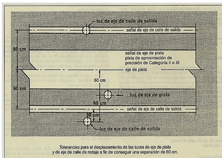
Figura 5-25. Desplazamiento de las luces eje de pista y de eje de calle de rodaje
