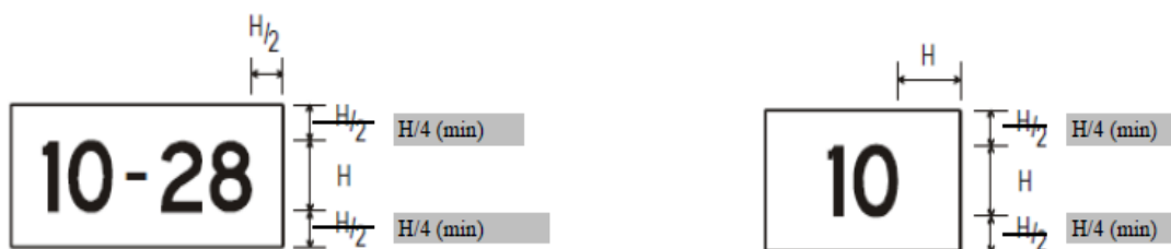
A. Letrero con dos designadores de pista
