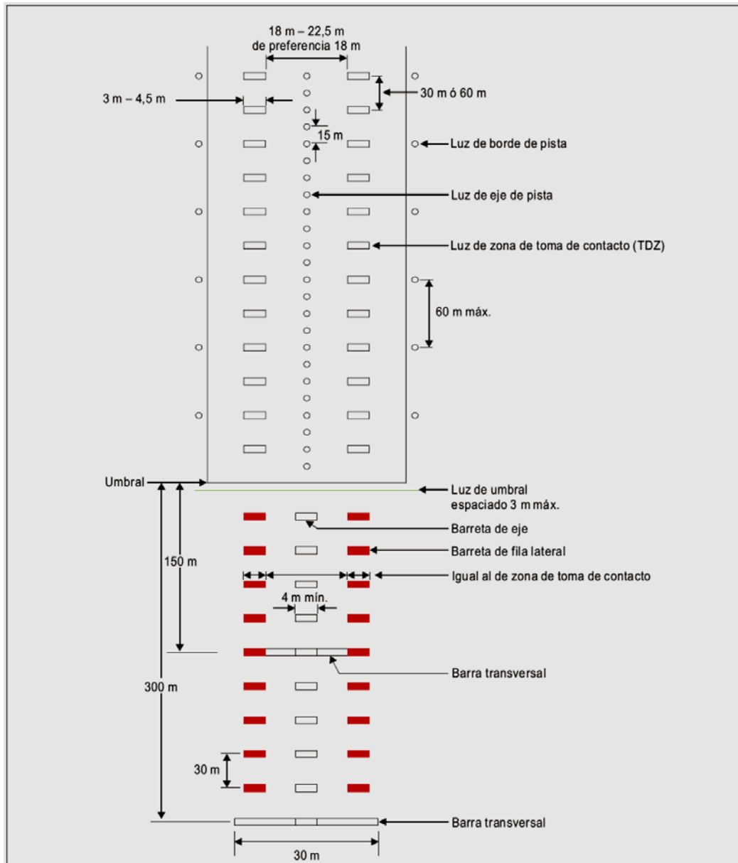
Figura 5-13. Iluminación de pista y de los 300m internos de la aproximación, en las pistas para aproximaciones de precisión de precisión de Categoría II y III
