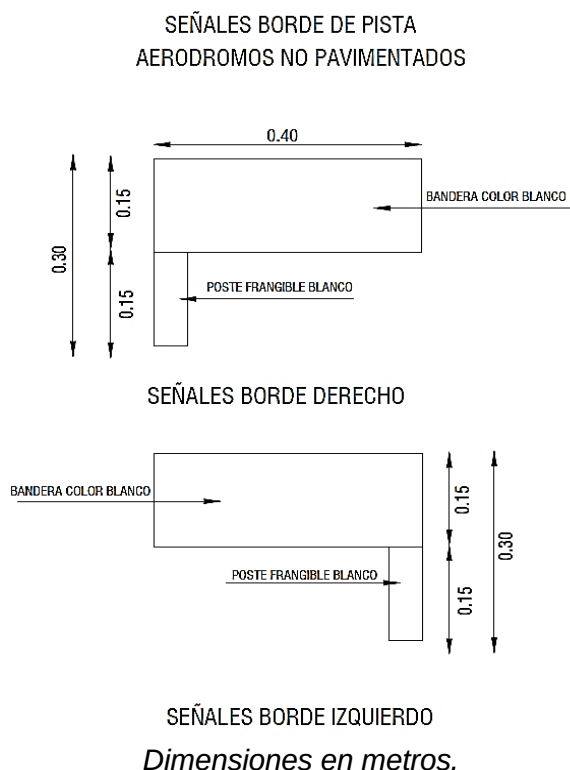
Figura 5-2. (E). Señal lateral (borde) para pista no pavimentadas.
