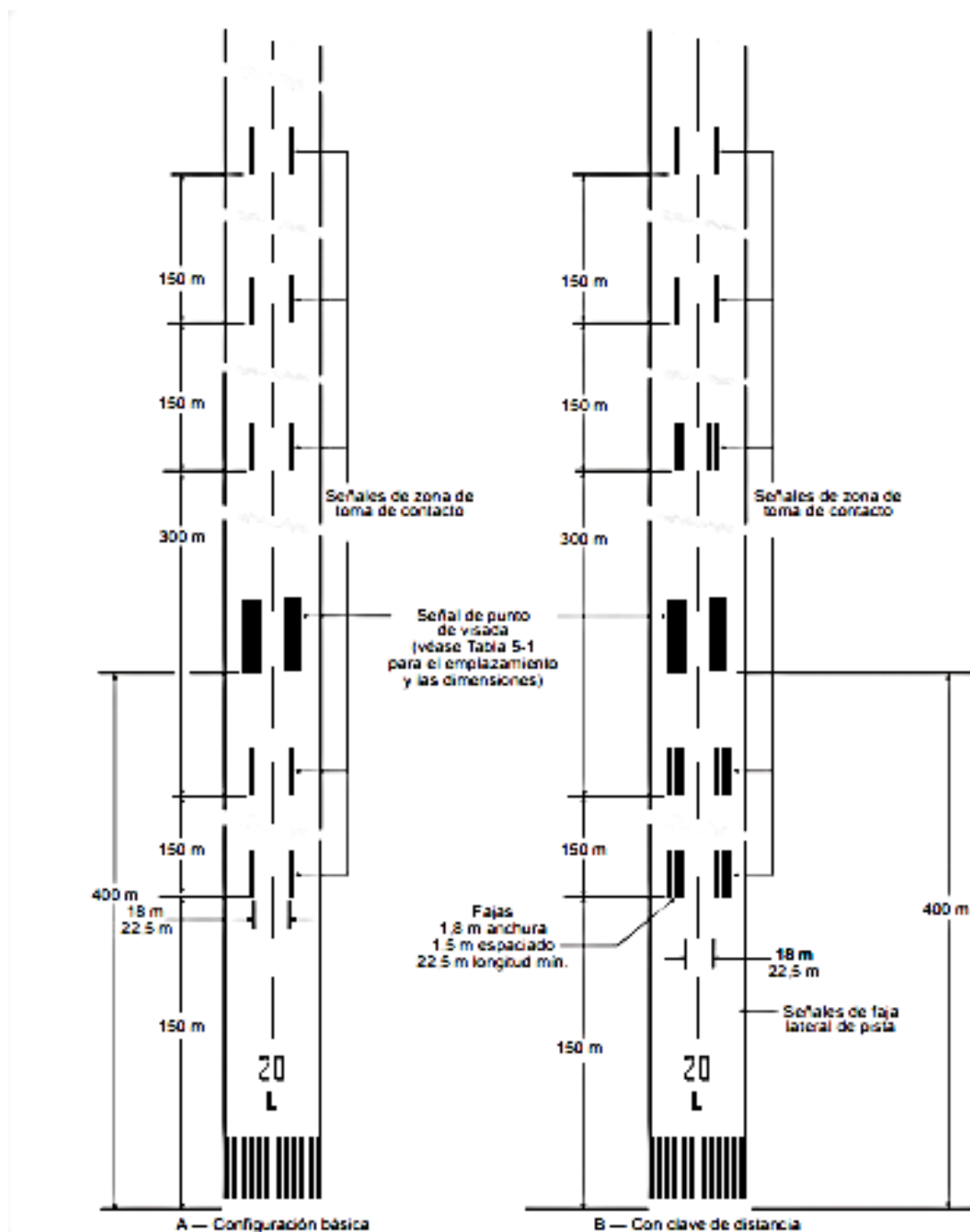
Figura 5-5. Señales de punto de visado y zona de toma de contacto
