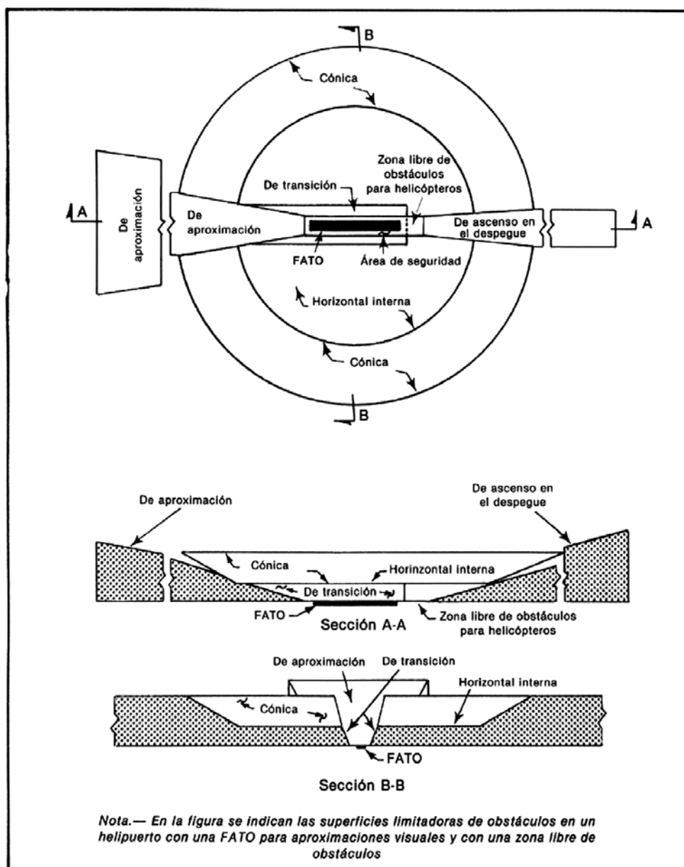
Figura 4-1H. Superficies limitadoras de obstáculos
