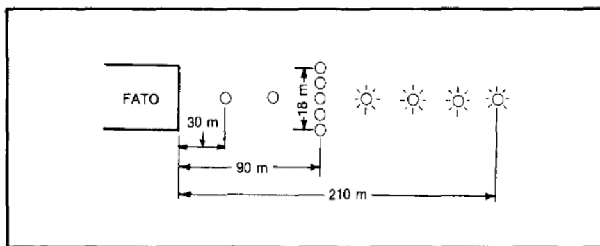
Figura 5-10H. Sistema de luces de aproximación
