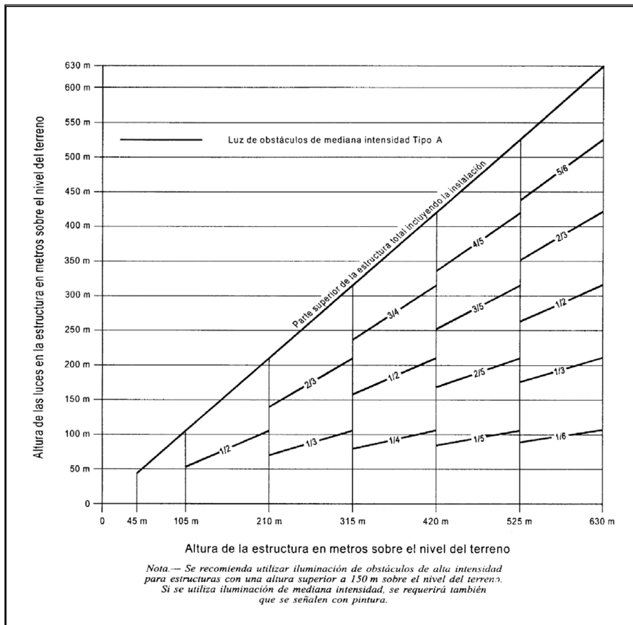
Figura A6 - 1. Sistema de iluminación de obstáculos con luces blancas de destello de mediana intensidad Tipo A
