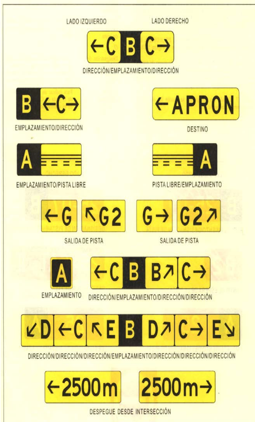
Figura 5-29. Letreros de información
