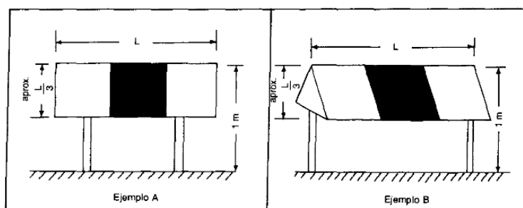
Figura 5-7H. Baliza de ruta de desplazamiento aéreo
